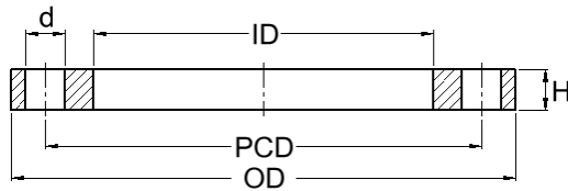
แหวนเหล็ก JIS/10 (BACKING RING JIS/10)
