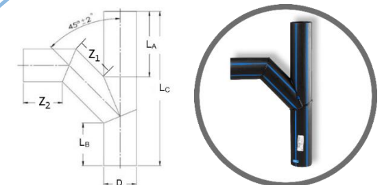
สามทาง 45° จาก (TEE WYES 45° PLUS)
